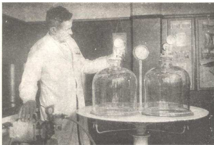
FIG. 1.—Dispositivo Farrar-Lepage-Gianotti.
